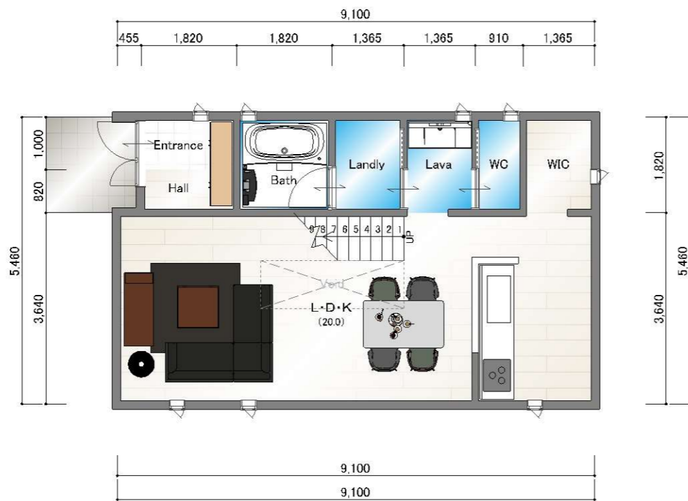
配置図 兼 1F平面図
